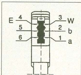
TAE-Steckerbelegung
